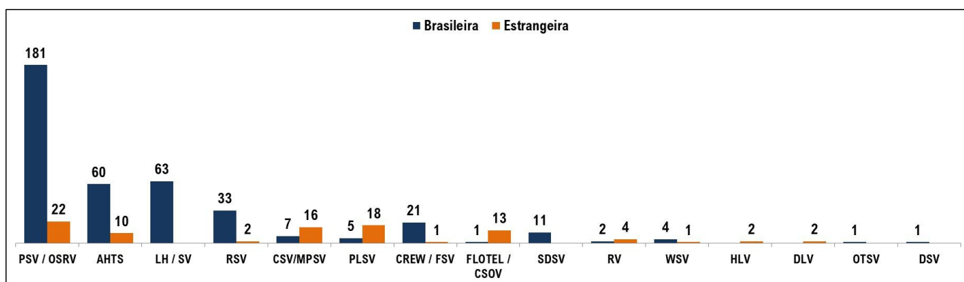
Gráfico 5 – Distribuição da frota total por tipo de embarcação e bandeira
